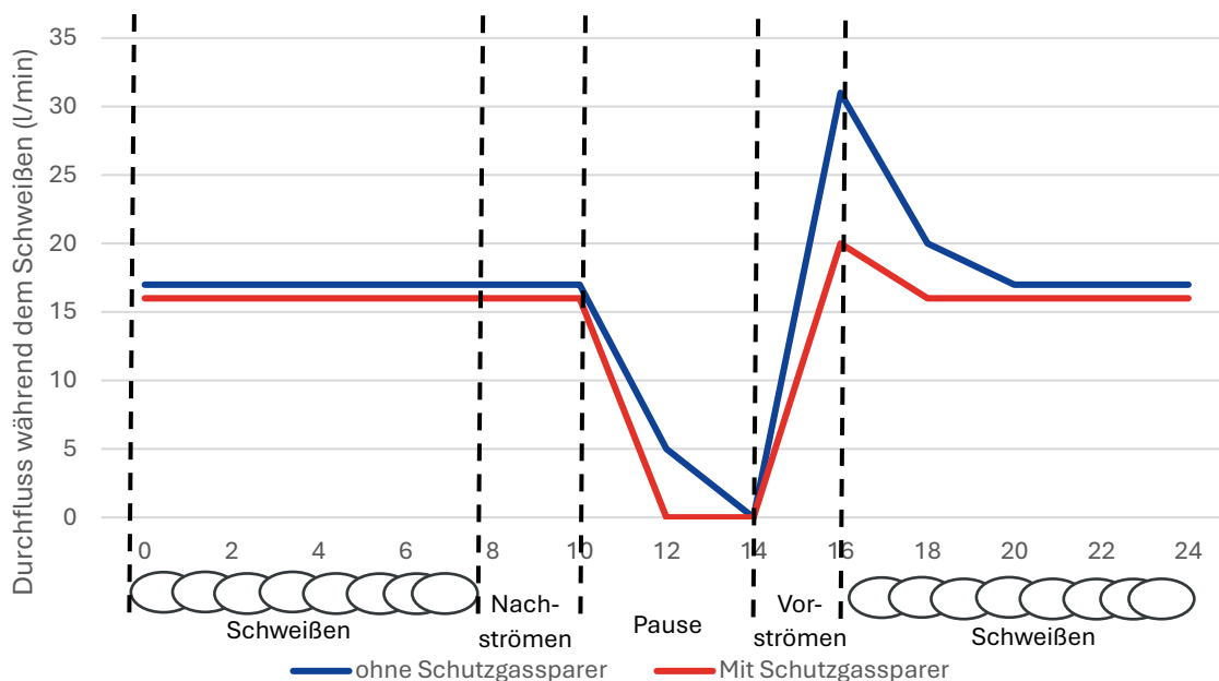
Prinzip eines Schutzgassparers
