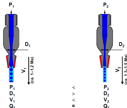
Standard-Schneiddüsen
